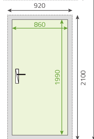
⑤ Kabinentür
